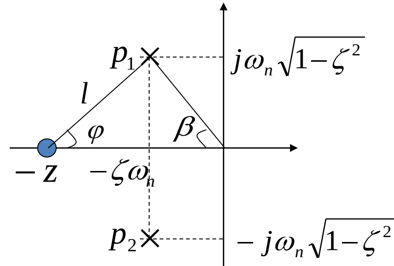
零极点分布图
