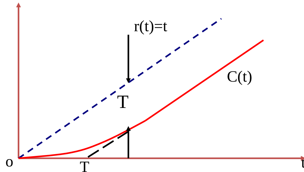
单位斜坡响应
