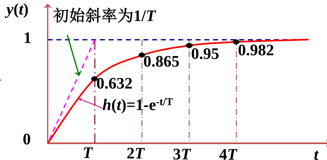
单位阶跃响应曲线
